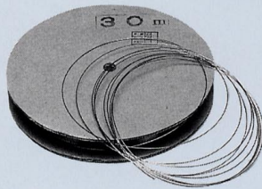
インバー線 IO 30M (φ0.5 mm x 長さ 30 m 巻)
