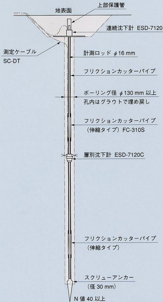
層別沈下計設置状態図
