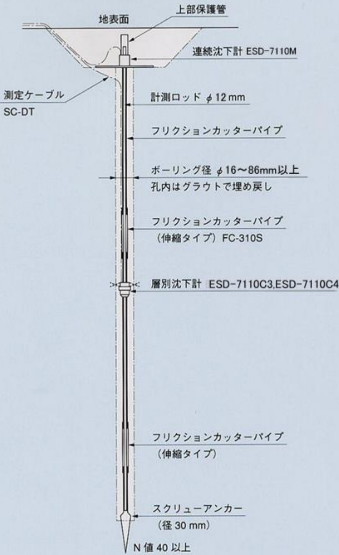
層別沈下計設置状態図
